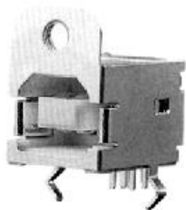
USB-2P-02
